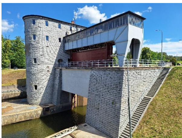
Ryc. 16. Śluza Kłodnica na Kanale Gliwickim
